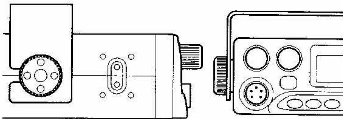
Рис. 4. Крепление радиостанции фиксаторами.
